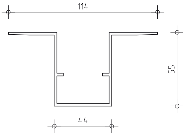
Hat section Art. 63803
